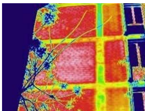
VERIFICA DISTACCO INTONACO
