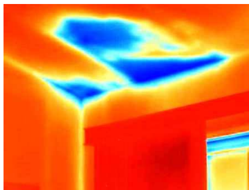
RILIEVO PERDITE SOLAI
